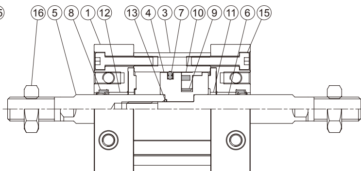
雙軸複動型
