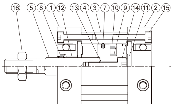
單軸複動型
