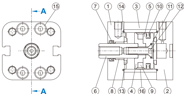
單軸複動型
