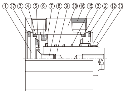
單動 押出型
