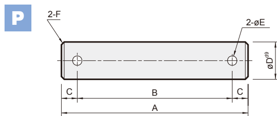
Y & I 型接頭用插銷尺寸表
